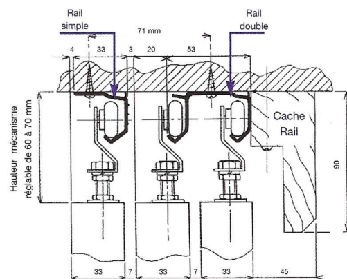
Si pose plafond avec jeu au sol 15 mm, prévoir: HAUTEUR PANNEAU = HAUTEUR (SOL/PLAFOND) - 90 mm
